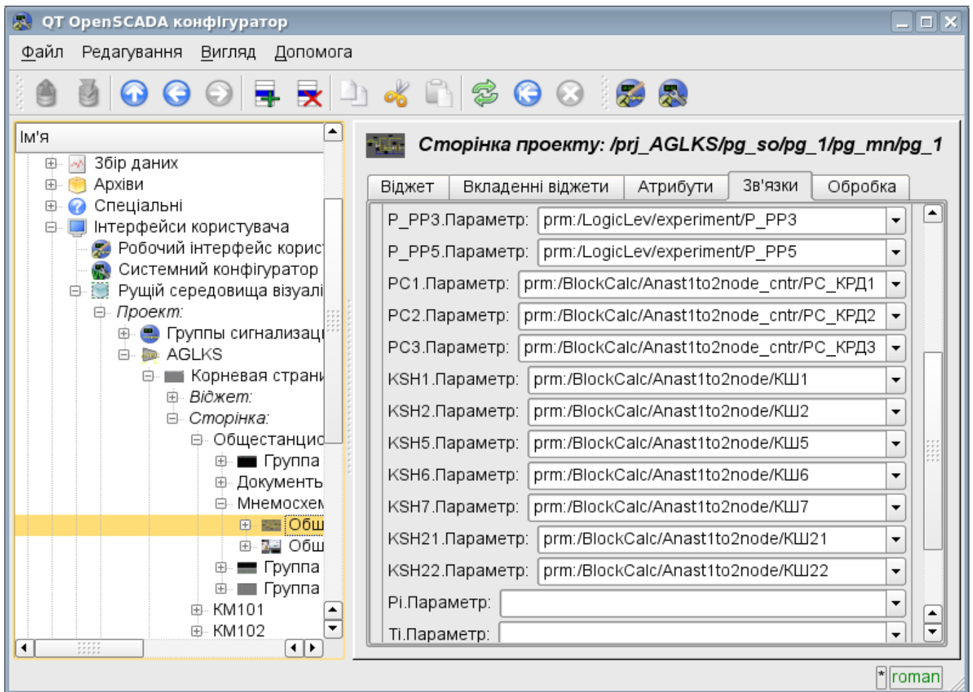
Рис. 3.7.d Вкладка "Связки" страницы конфигурации контейнера виджетов, включающего виджеты со связями.
