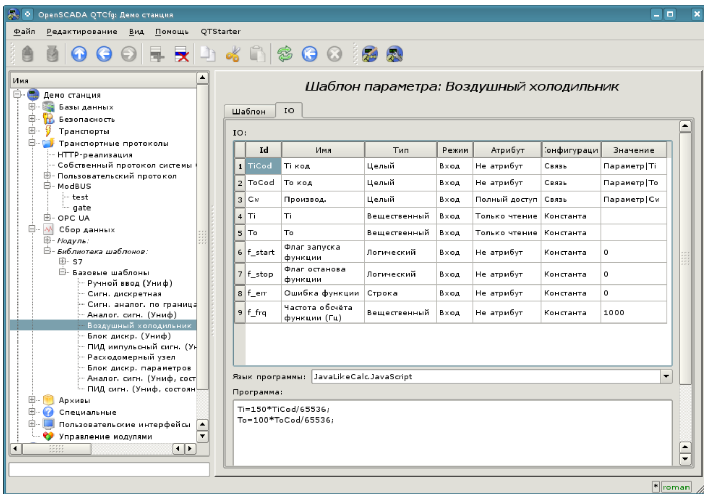
Рис. 4.2.2. Вкладка "ИО" страницы конфигурации объекта шаблона.
