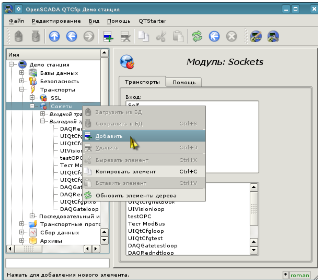
Рис. 4.1.4. Добавление исходящего транспорта в модуле "Sockets" подсистемы "Транспорты".
