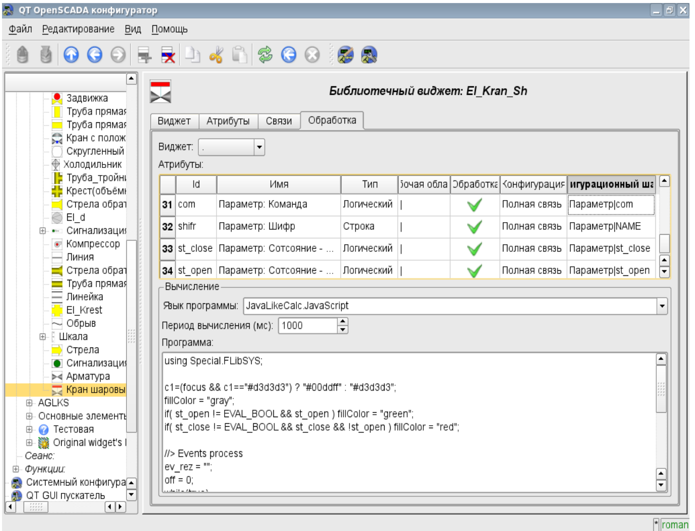
Рис. 3.7.а Вкладка "Обработка" страницы конфигурации виджета.
