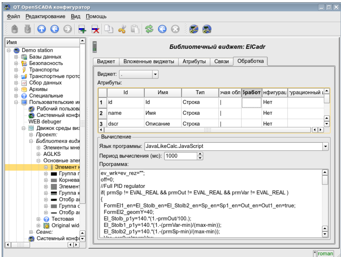
Рис.4.10 Вкладка обработки визуальных элементов.
